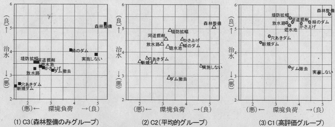
図-4 各洪水リスク軽減策の「治水効果」と「環境負荷」に関する評価プロット
