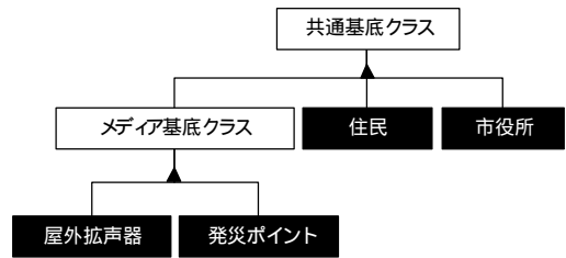
図 - 1 プログラムのクラス構造
